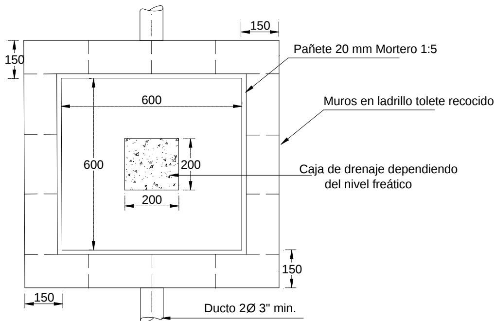
PLANTA CAJA Y MUROS
