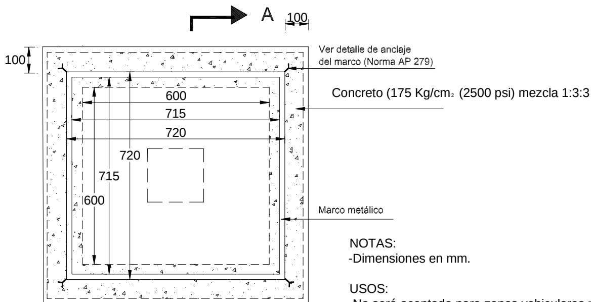
PLANTA CAJA Y MUROS
