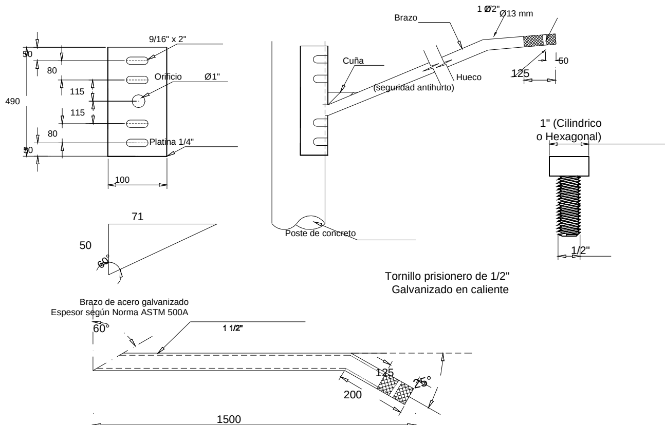
FIGURA 8. Soporte para luminaria peatonal 9000 mm. (Este soporte es para vías peatonales y ciclovías en postes de 12 y 14 m)
