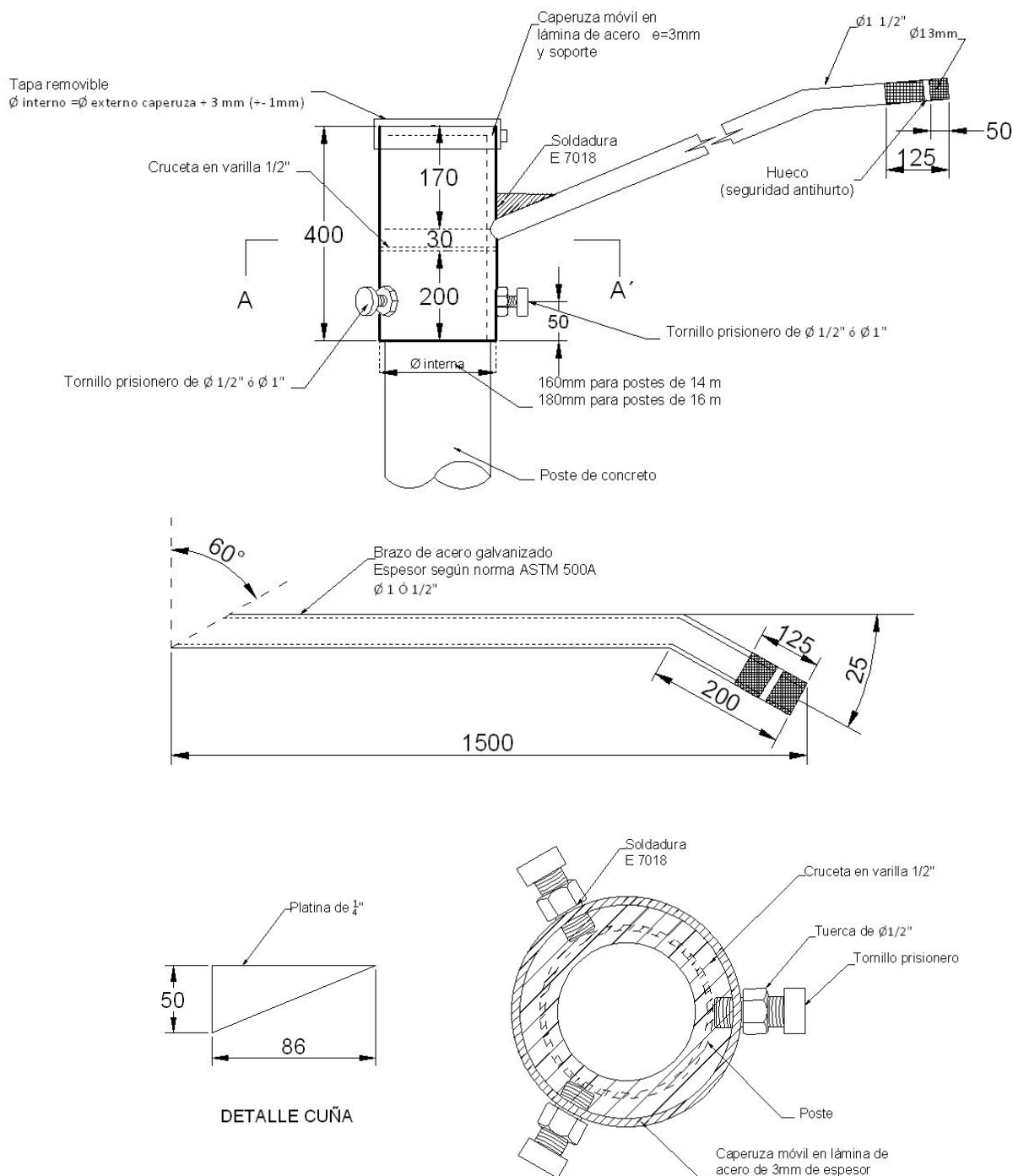
FIGURA 5. Soporte sencillo para luminaria
